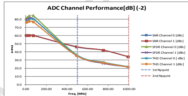
(d) ADC SNR/SFDR/THD vs frequency (DC version)
